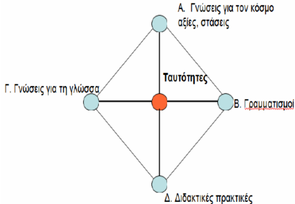
Σχήμα 3. Ρόμβος και ταυτότητες
